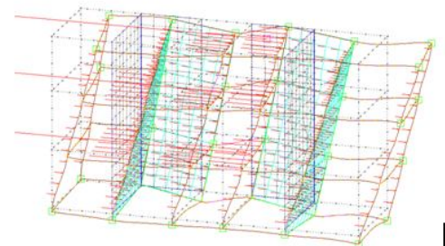
Modello della struttura soggetta a carichi orizzontali portata al collasso - Scuola Nicholas Green - Corpo 3
