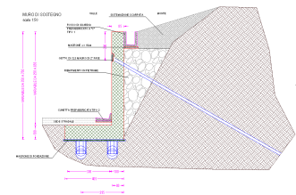
Sezione Muro di sostegno
